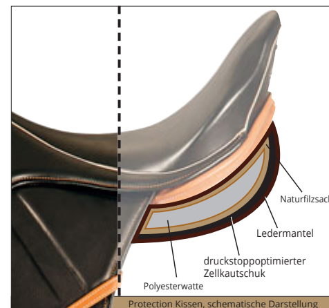
Protection Kissen, schematische Darstellung
